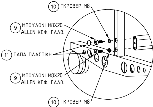
ΛΕΠΤΟΜΕΡΕΙΑ Β
