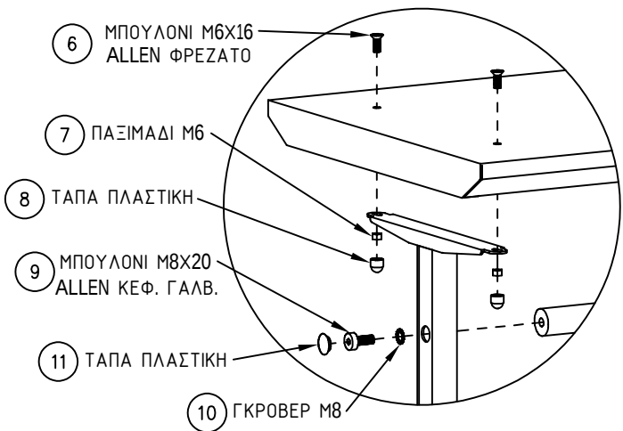
ΛΕΠΤΟΜΕΡΕΙΑ Α
